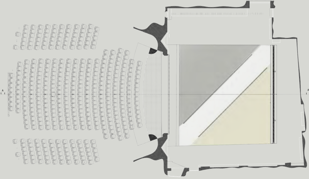
Low Plan 1:100
