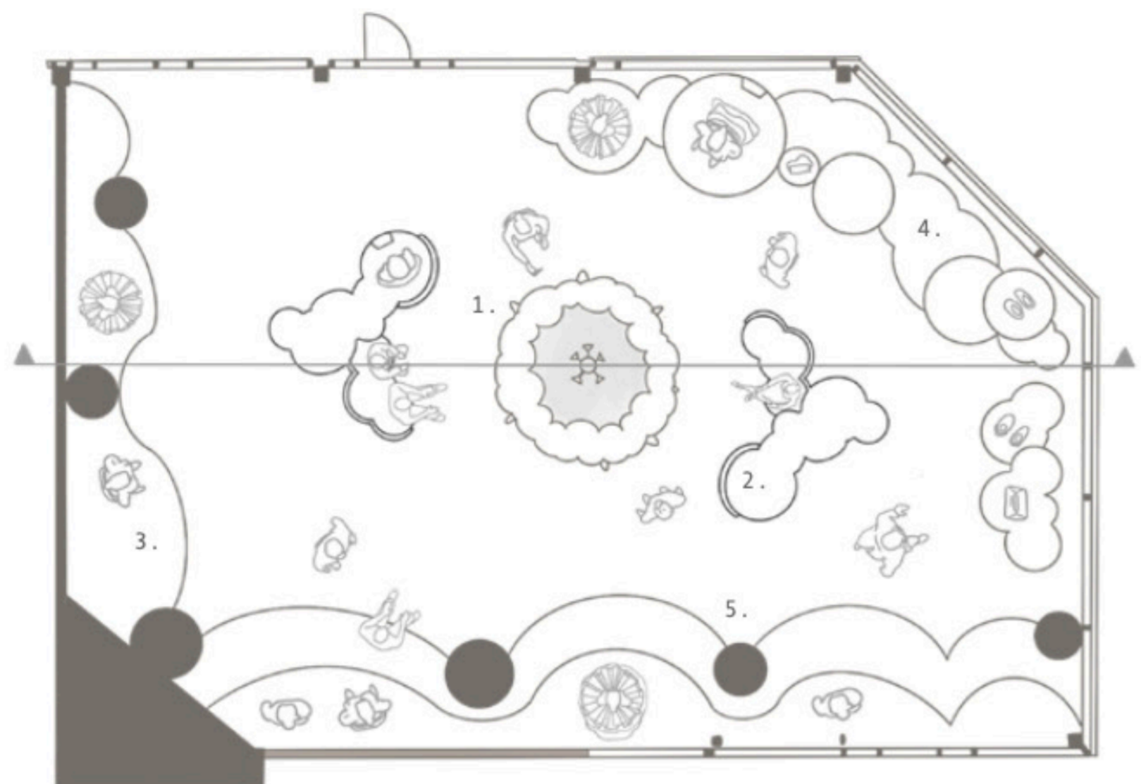
Floor plan @A3 1:100
